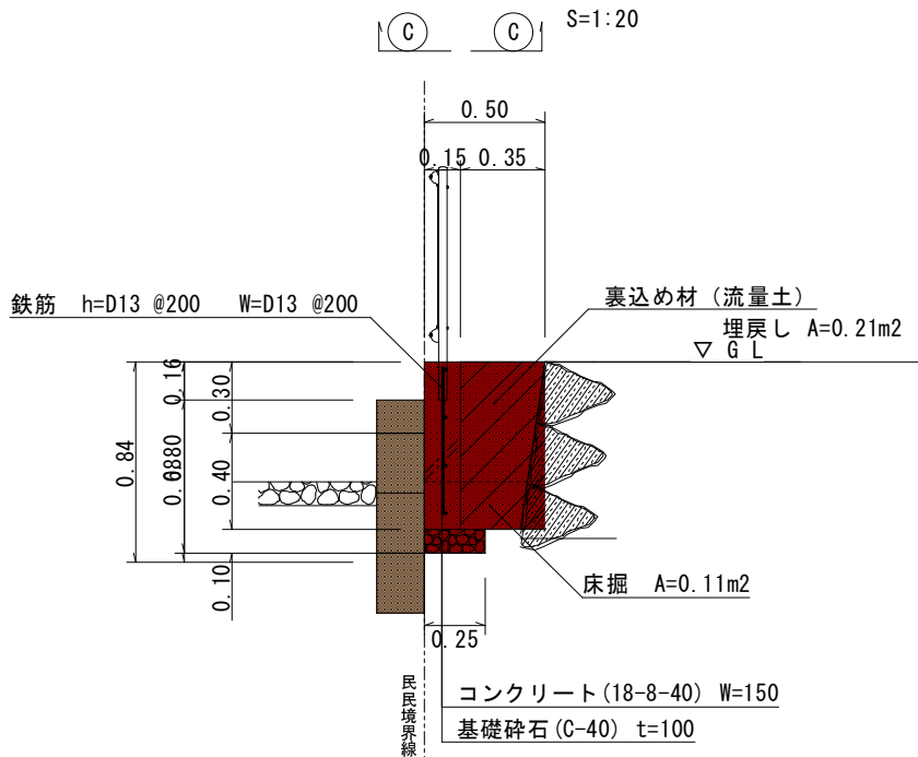
石 積 み 詳 細 図
