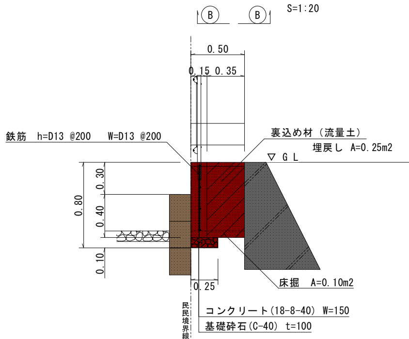
現場打ち擁壁詳細図
