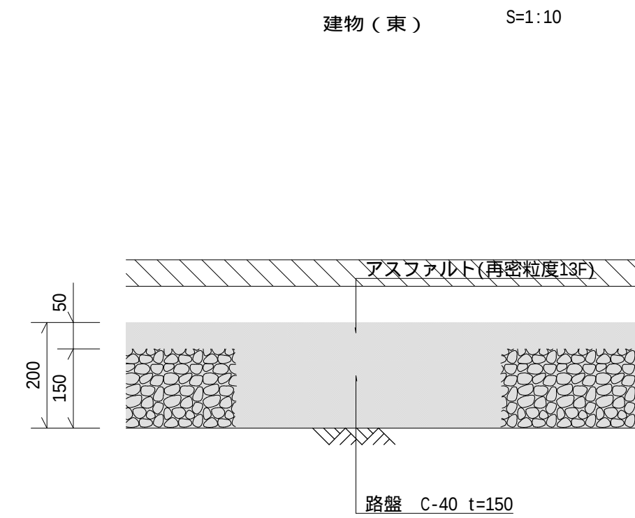
アスファルト舗装標準図
