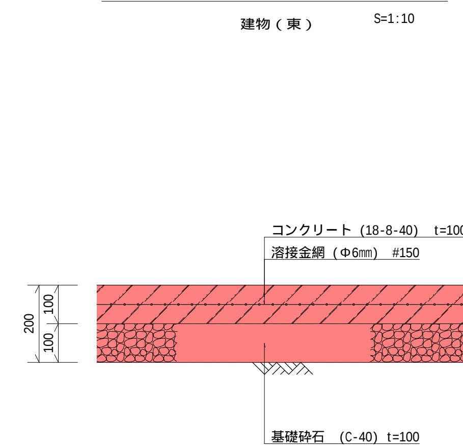
コンクリート詳細図
