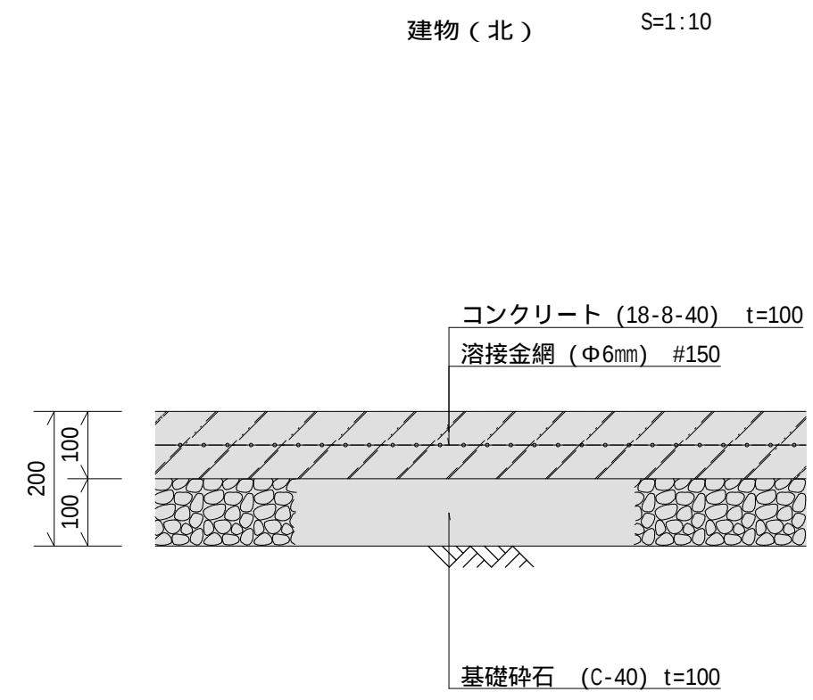
コンクリート詳細図
