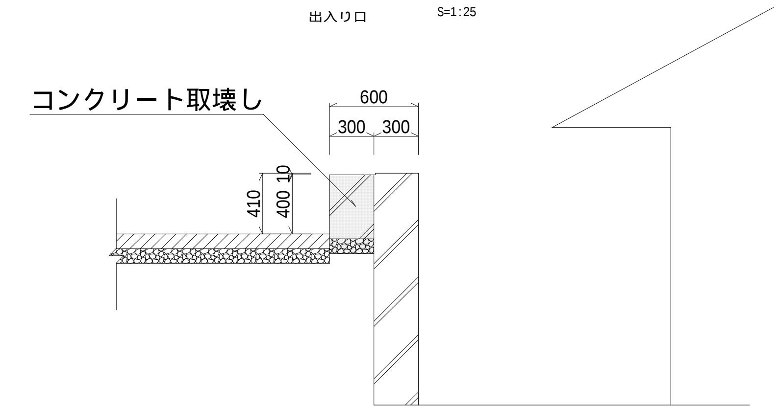
擁壁背面詳細図
