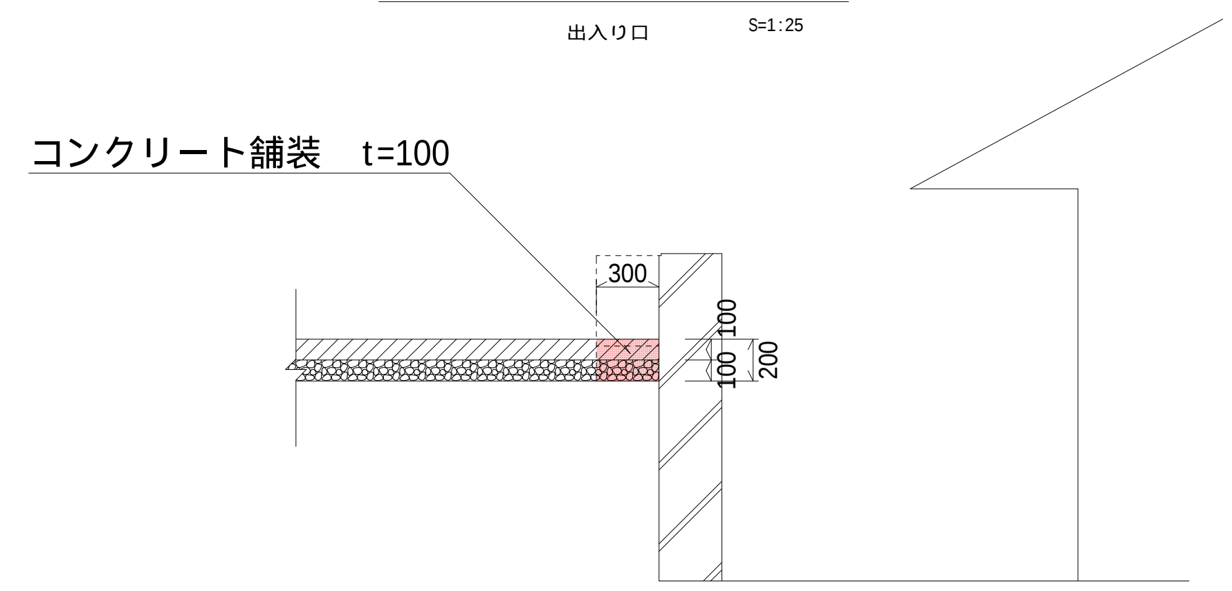
擁壁背面詳細図
